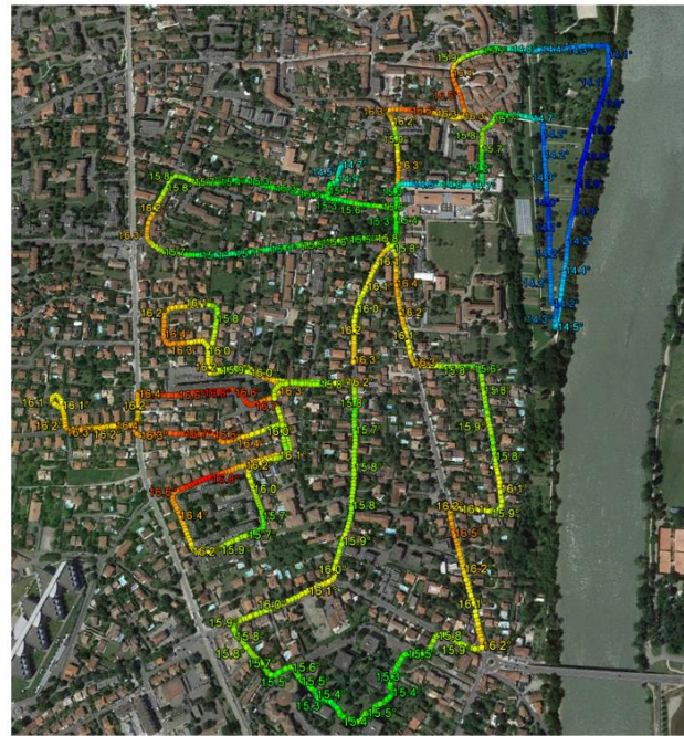
Figure 3.3.i. Variabilité du climat urbain : caractérisation de l'ICU moyen (4°C) à Toulouse grâce aux données de la campagne de mesures scientifiques CAPITOUL (à gauche) ; variations de la température de l'air (4°C) dans un quartier périurbain (Blagnac) caractérisées dans le cadre du PIRVE « Hétérogénéités climatiques, paysagères et sociales ». (sources : Pigeon et al. 2007 ; Haouès-Jouve et al., sous presse)
