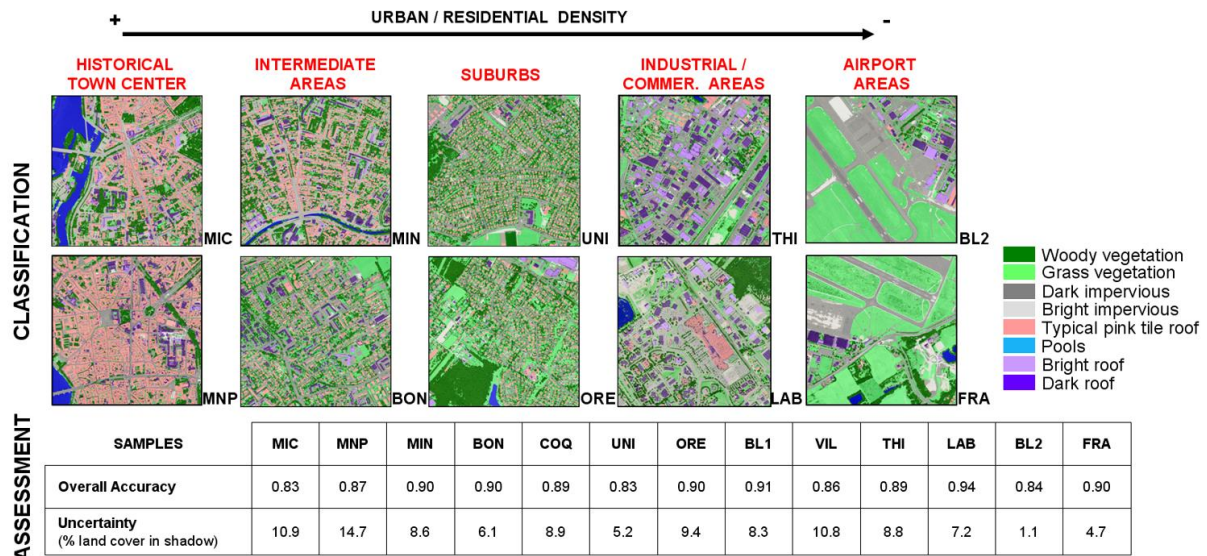
Figure 3.3.a. Classifications des types d'occupation des sols pour les stations : MIC (Saint-Michel), MNP (Monoprix), MIN (Minimes), BON (Bonnetoy), UNI (Union), ORE (Saint-Orens), THI (zone Thibault), LAB (Labège), BL2 (Blagnac 2) et FRA (Francazal) et leur évaluation. (Source : Houet and Pigeon, 2011)
