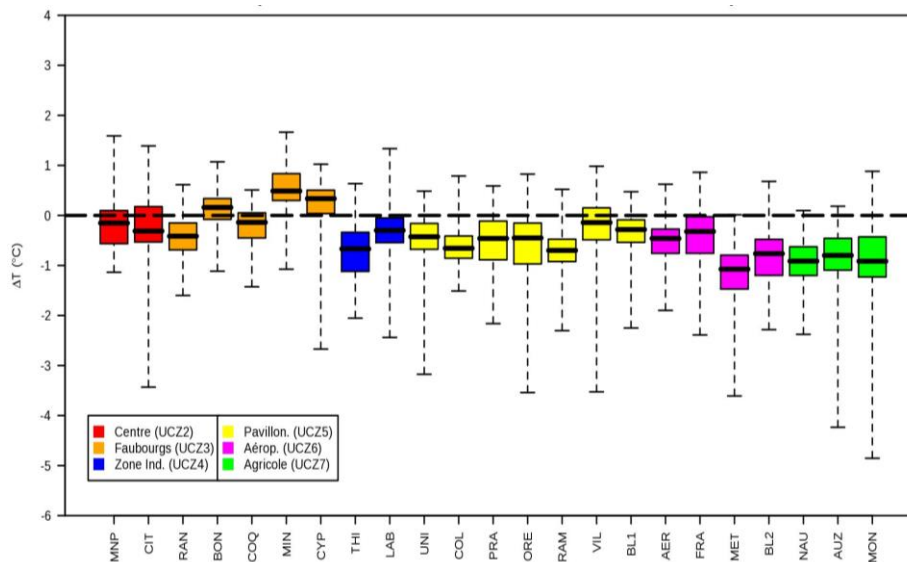
Figure 3.3.d. Boîtes à moustaches montrant les différences de températures des stations CAPITOUL par rapport à la station de référence (MIC) située en centre-ville en situation estivale et de jour. (Source : Houet and Pigeon, 2011)
