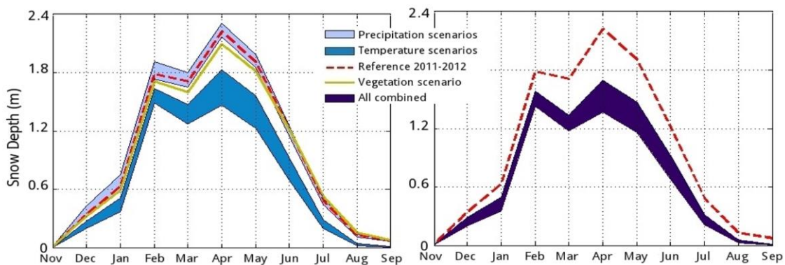
Figure 3.4.l. Impact respectif (gauche) et combiné (droite) des variables d'entrée de Snowmodel (T°, Pmm, Changements de végétation) par rapport à la situation de référence de 2011-12. (Source : Sczcypta et al. 2015)
