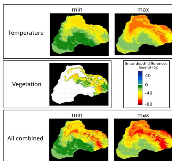
Figure 3.4.m. Impact respectif et combiné des variables d'entrée de Snowmodel (T°, Pmm, Changements de végétation) de façon spatialisée par rapport à la situation de référence de 2011-12. (Source : Sczcypta et al. 2015)
