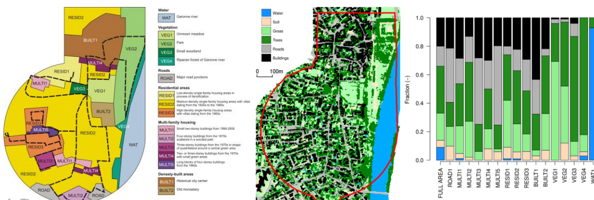
Figure 3.3.f. A gauche : Unités paysagères urbaines identifiées par une approche experte au sein du l'UCZ5 BLA (projet CAPITOUL). A droite : classification des types d'occupation des sols et composition des unités paysagères. (Source : Lemonsu et al. Submitted)
