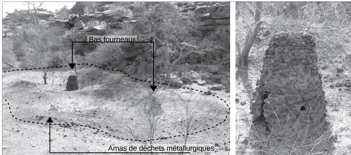
Fig. 34. Site de réduction N2.
