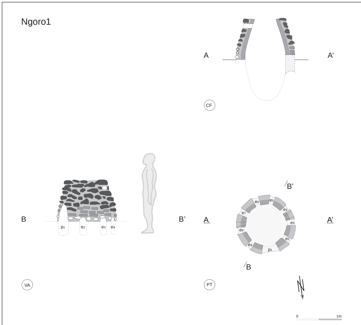
Annexe 8. Plan et coupes du bas fourneau du site Niongono 2A, PT : plan transversal ; V : vue ; CS : coupe.
