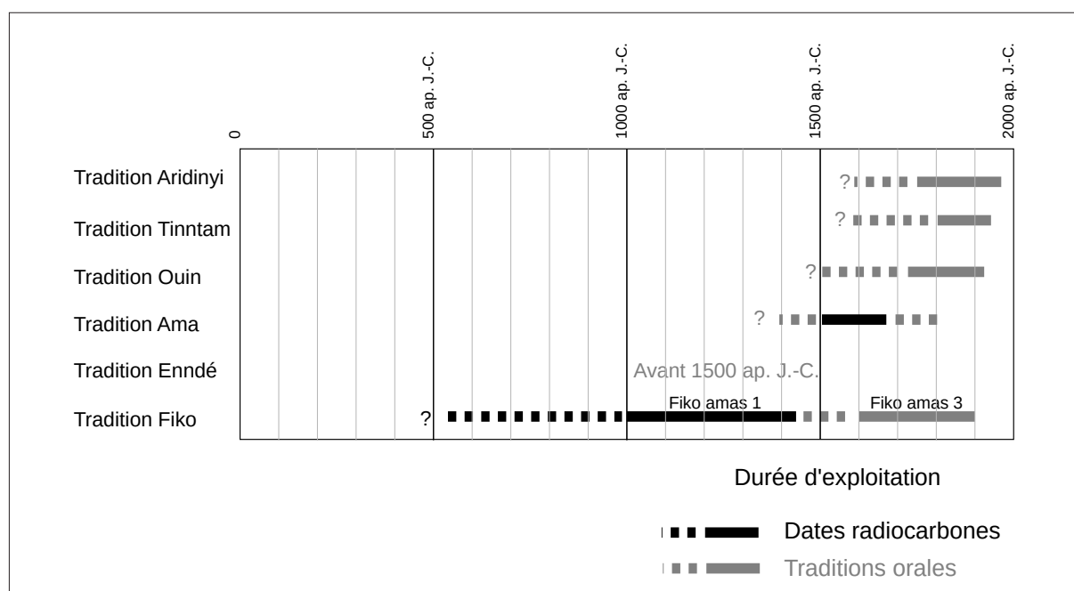
Fig. 64. Synthèse chronologique de la production du fer par tradition sidérurgique.
