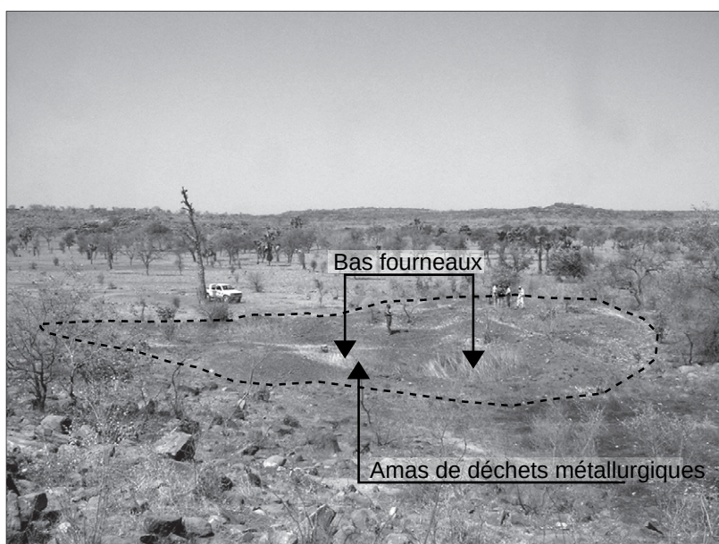
Fig. 31. Site de réduction B4. Smelting site B4.
