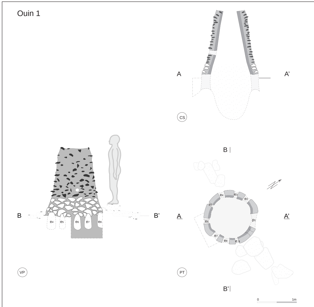
Annexe 4. Plan et coupes du bas fourneau du site Ouin 1, PT : plan transversal ; VP : vue postérieure ; CS : vue sagittale.
