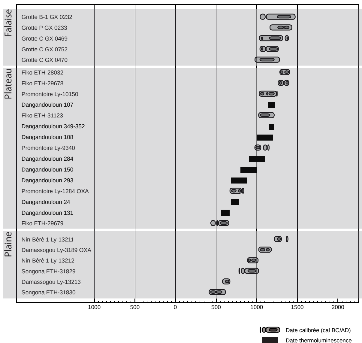
Fig. 68. Dates radiocarbone liées aux occupations et aux sites sidérurgiques dogon.
