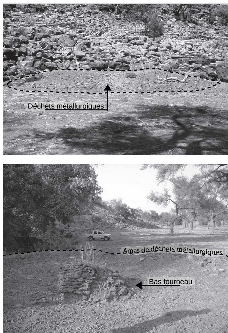
Fig. 28. Sites de réduction O3 et O4. Smelting sites O3 and O4.
