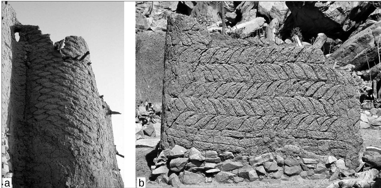
Fig. 37. a : Grenier du village Ouin ; b : Brique d'une maison de Dogo.
