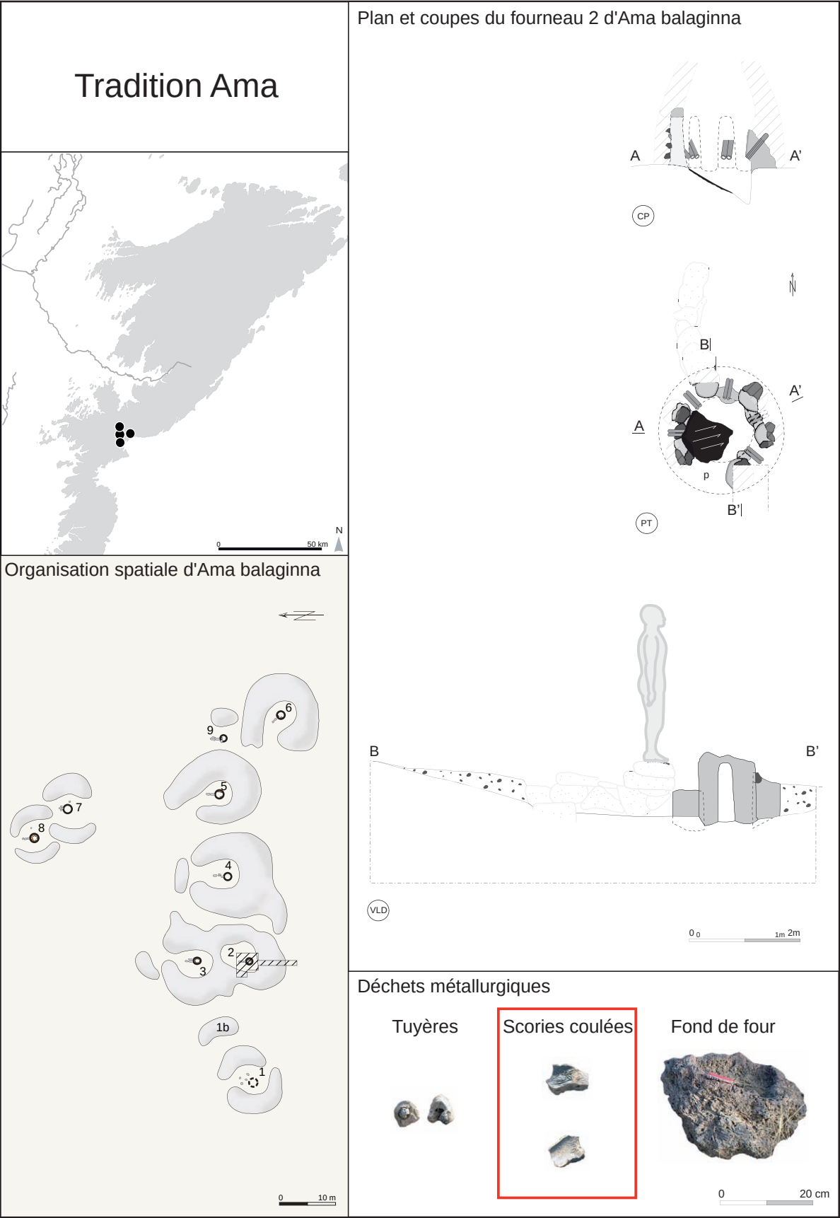
Pl. 7. Caractéristiques principales de la tradition Ama (Légende: Pl. 11–12, Annexe 3 ). Main characteristics of the Ama tradition (Key: Pl. 11–12, Annexe 3).
