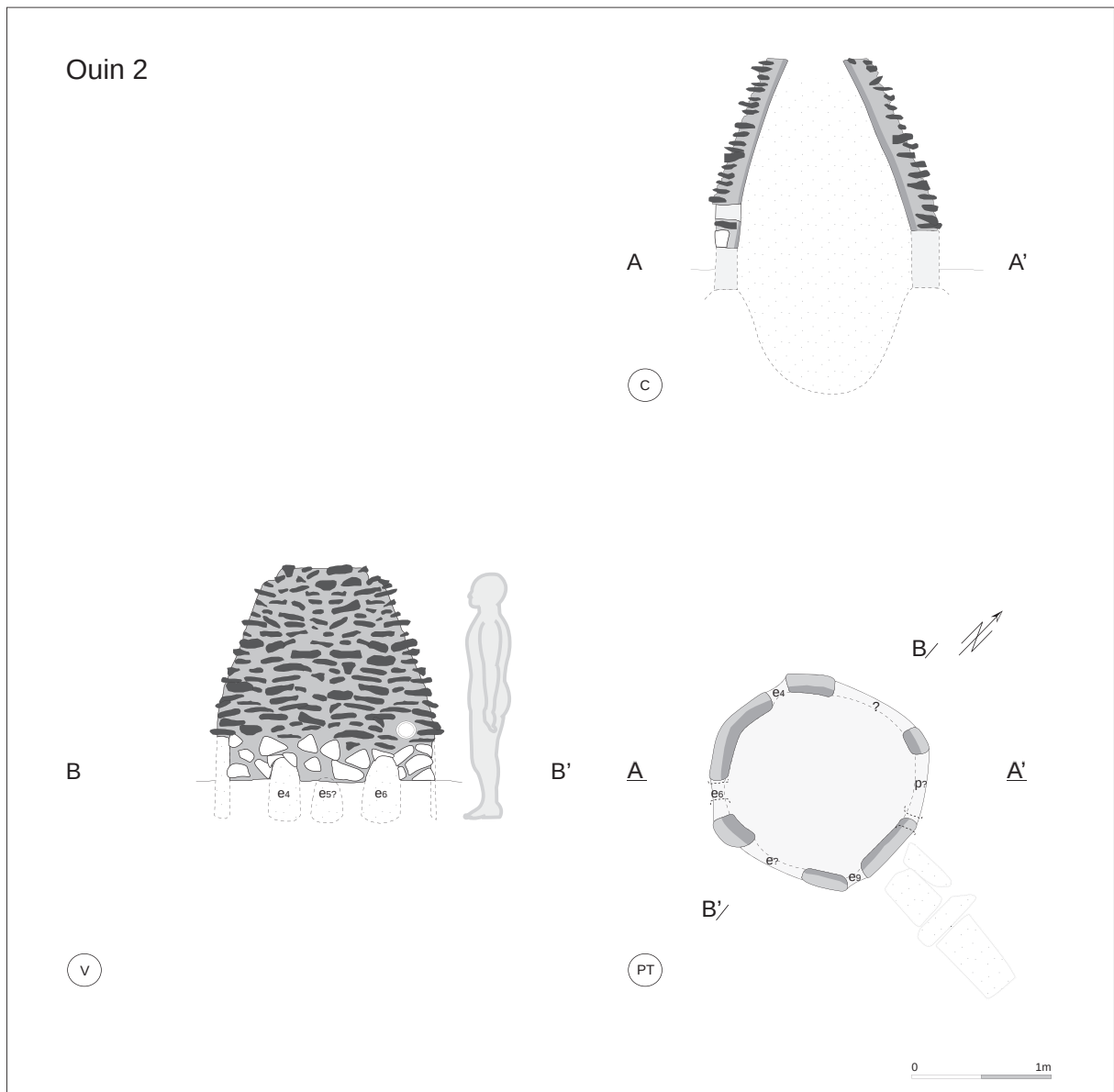
Annexe 5. Plan et coupes du bas fourneau du site Ouin 2, PT : plan transversal ; V : vue ; C : coupe.
