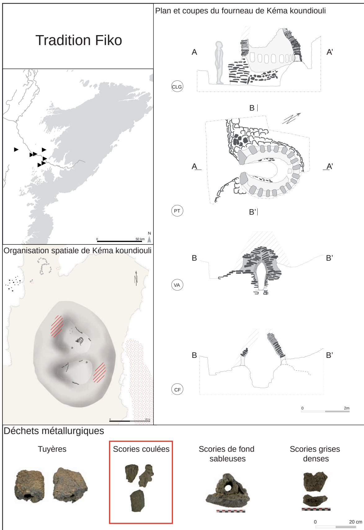
Pl. 6. Caractéristiques principales de la tradition Fiko (Légende: Pl. 11–12, Annexe 3 ).
