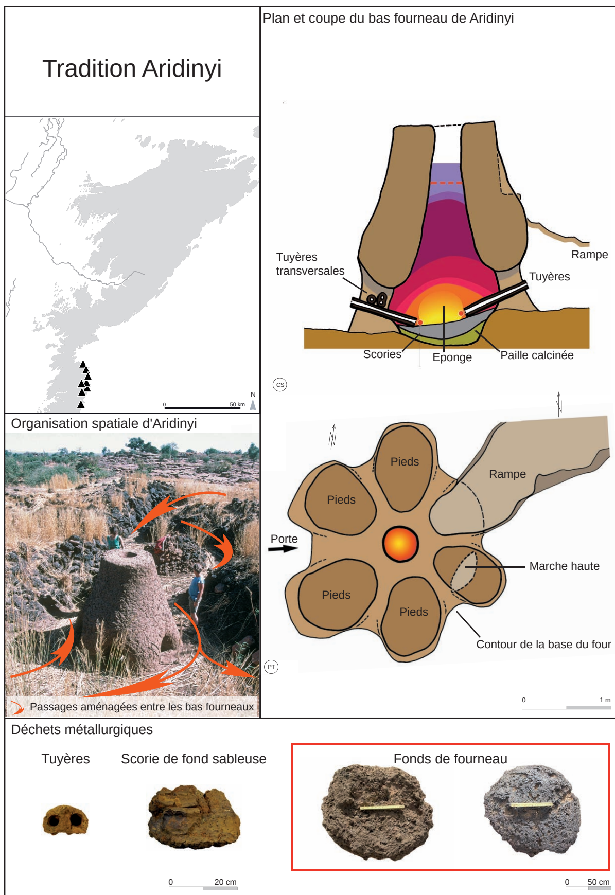
Pl. 9. Caractéristiques principales de la tradition Aridinyi (Dessins de E. Huysecom, DESCOEUDRES et al. 2001 : planches II-2 et IV). Main characteristics of the Aridinyi tradition (drawing by E. Huysecom, DESCOEUDRES et al. 2001: planches II-2 et IV).
