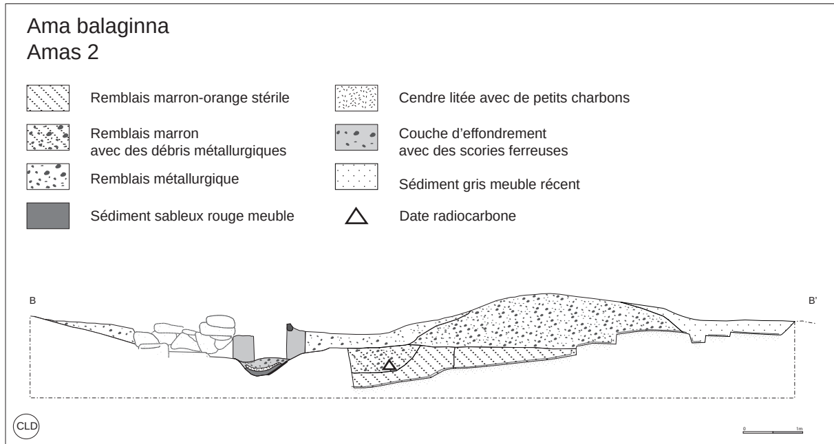
Fig. 48. Coupe postérieure du bas fourneau 2 du site Ama balaginna.
