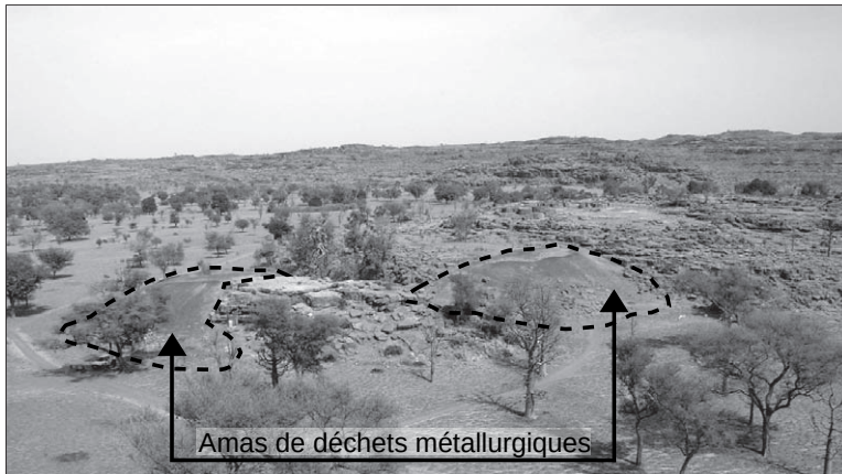
Fig. 33. Site de réduction N1. Smelting site N1.
