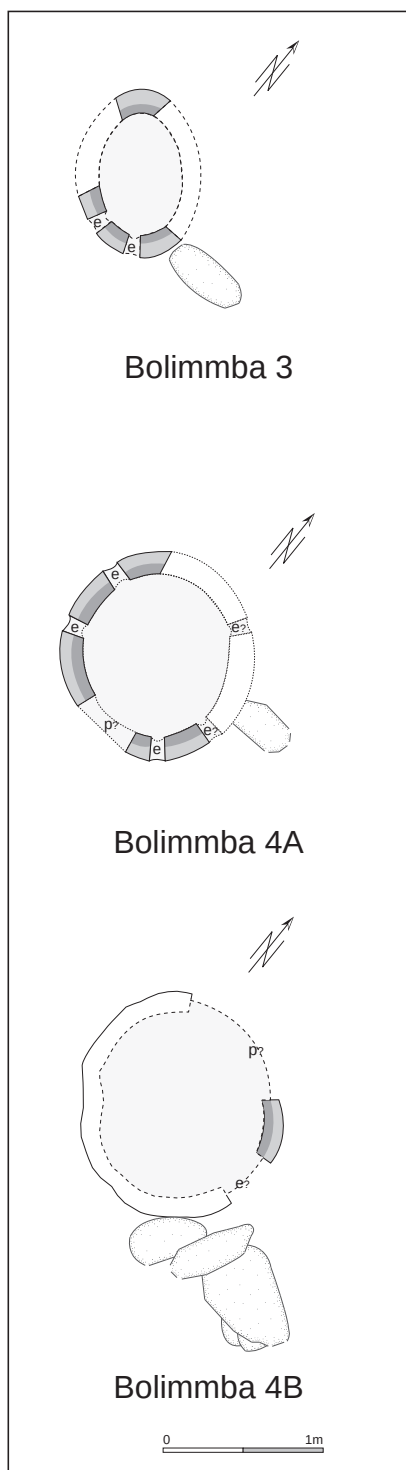
Annexe 6. Plans transversaux des bas fourneaux Bolimmba 3, 4A et 4B. Transverse planes of the bloomery furnaces Bolimmba 3, 4A et 4B.
