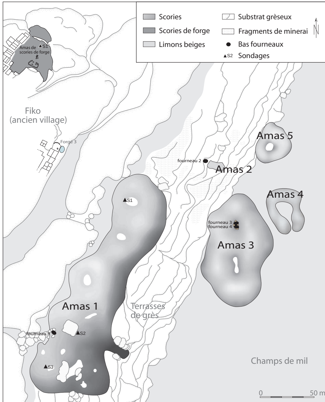
Fig. 39. Relevé topographique des vestiges sidérurgiques anciens de Fiko (Dessin de S. Perret, HUYSECOM et al. 2004 : 54).
