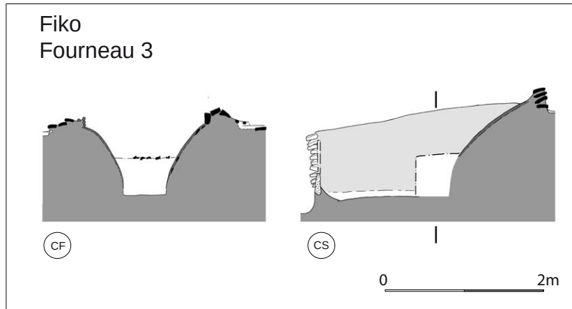
Annexe 9. Coupes du bas fourneau 3 de l'amas 3 de Fiko (Dessin de S. Perret, HUYSECOM et al. 2006 : 145).
