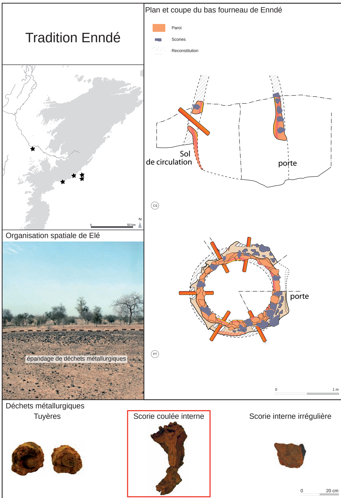
Pl. 10. Caractéristiques principales de la tradition Enndé (Dessins de S. Perret).
