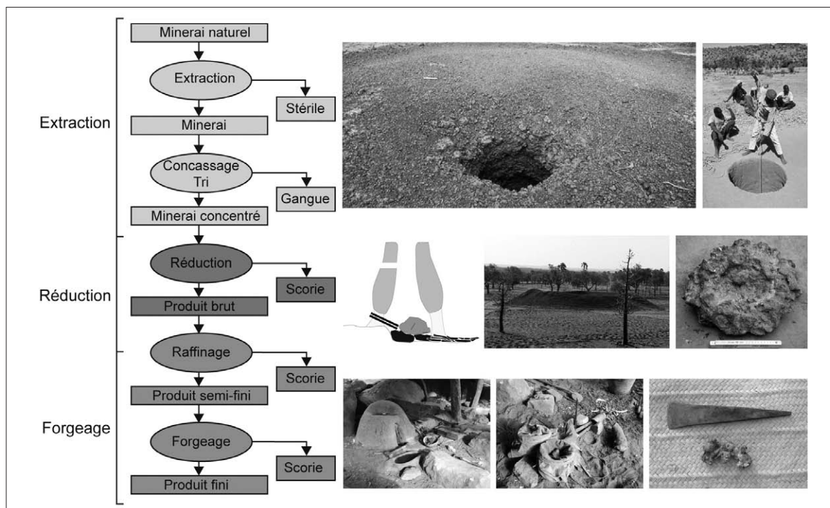
Fig. 1. Schéma général de la chaîne opératoire de la sidérurgie selon la méthode directe de réduction (d'après GSAF 1997 : 8). General scheme of the chain of operations of the iron production using the bloomery process (from GSAF 1997: 8).
