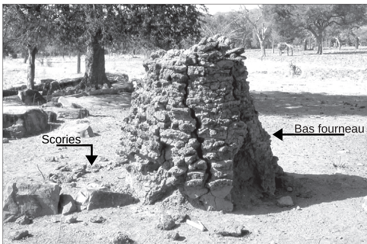
Fig. 27. Bas fourneau O2. Bloomery furnace O2.
