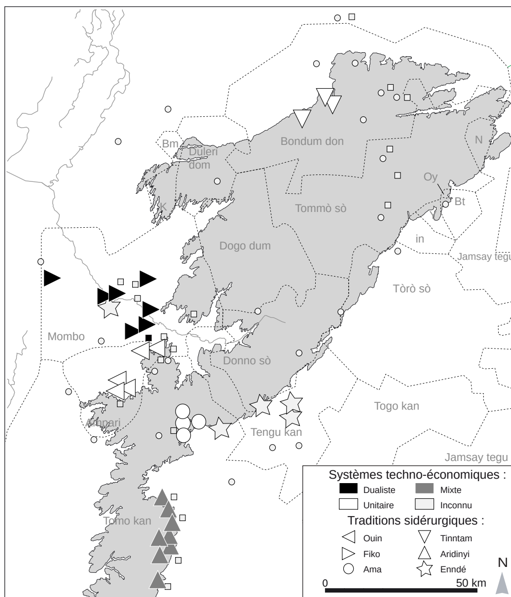
Fig. 67. L'organisation techno-économique des traditions sidérurgiques du pays dogon.
