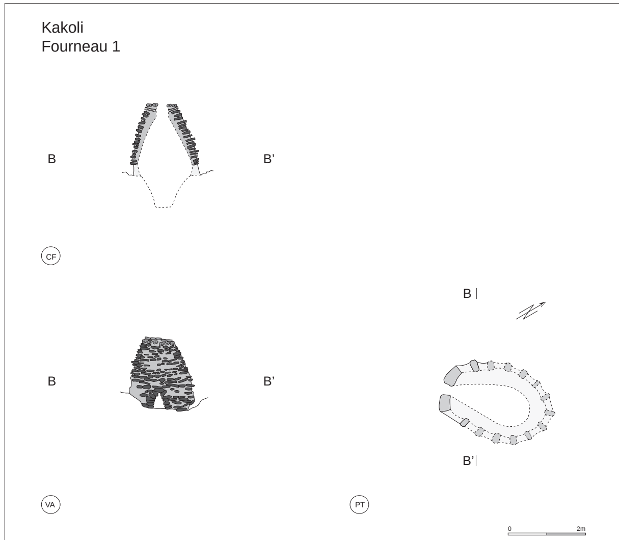
Annexe 10. Plan et coupes du bas fourneau du site Kakoli, PT : plan transversal ; VA : vue antérieure ; CF : coupe frontale.
