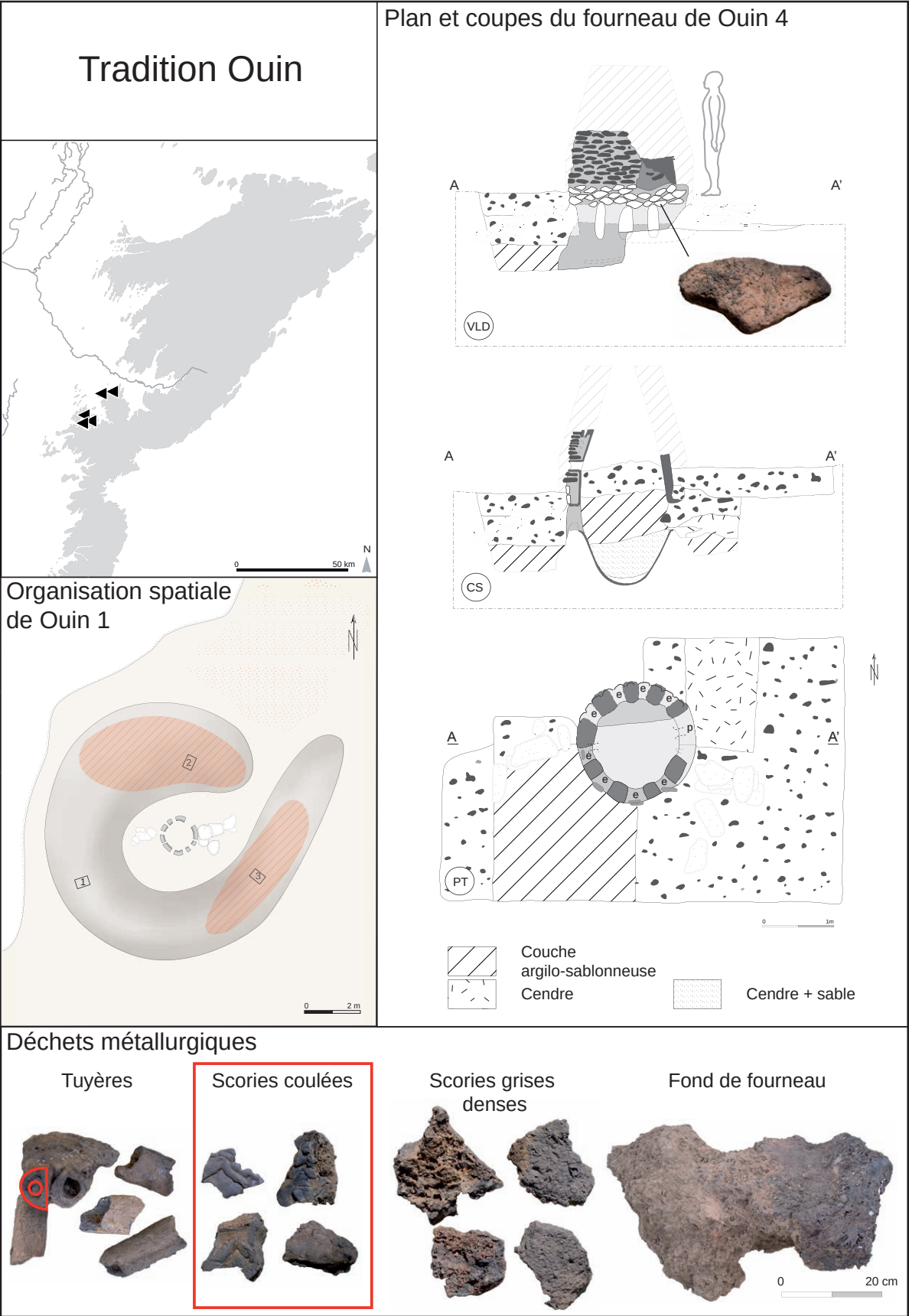
Pl. 5. Caractéristiques principales de la tradition Ouin (Légende: Pl. 11–12, Annexe 3 ).
