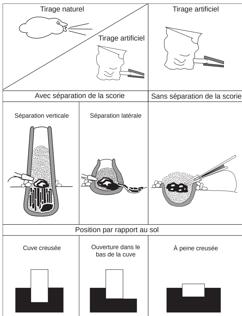
Fig. 6. Classification simplifiée des bas fourneaux (d'après SERNEELS 1998 : 16).
