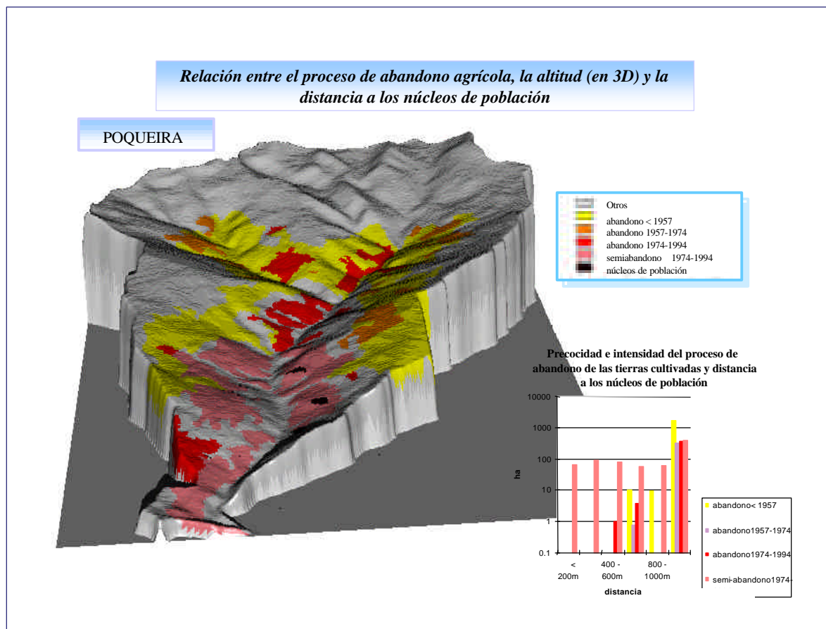
Figura nº15 - Abandono agrícola del valle de Poqueira, altitud (en 3D) y distancia a los núcleos de población
