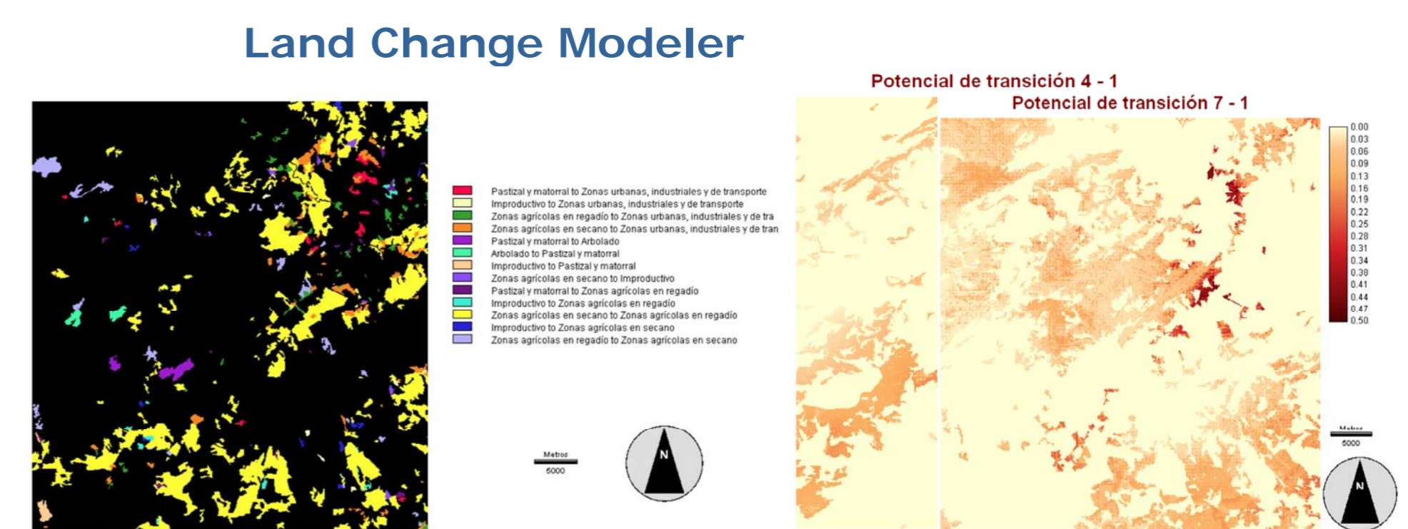
Figura 5. Transiciones 1990-2000 (<5000 píxeles)
